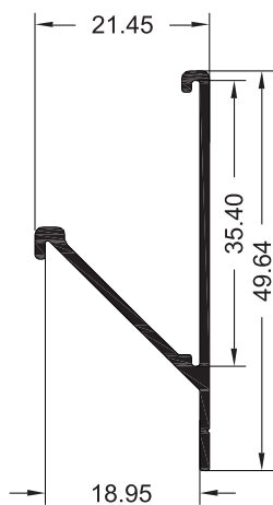
Perfil Y
