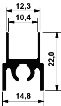
TUBO 3/8
