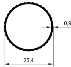
TUBO CANALETADO 1'
