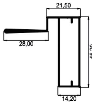
TUBO CANALETADO 1'
